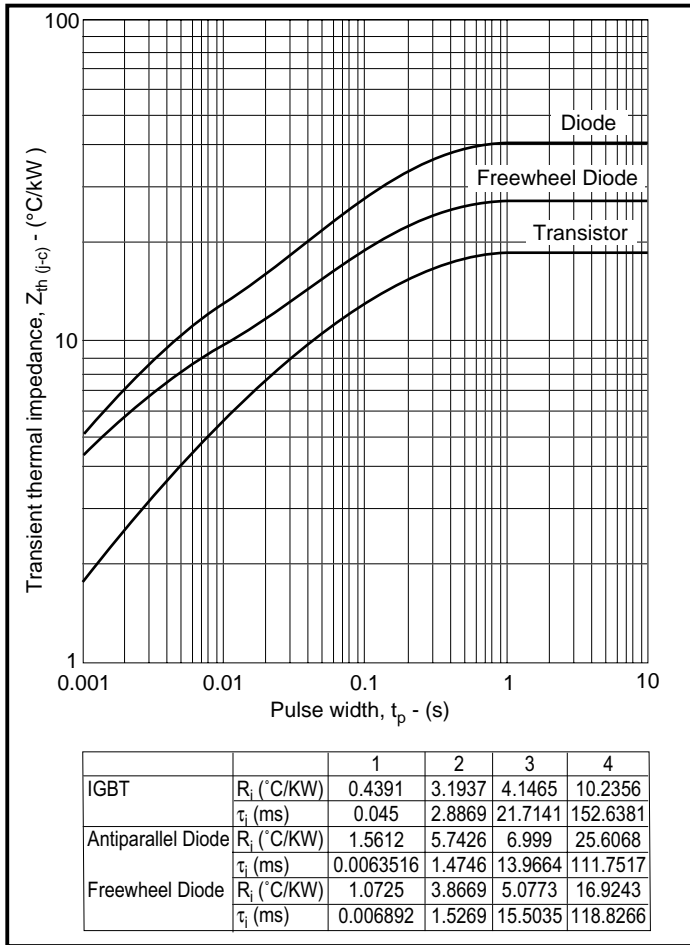
Fig. 13 Transient thermal impedance
